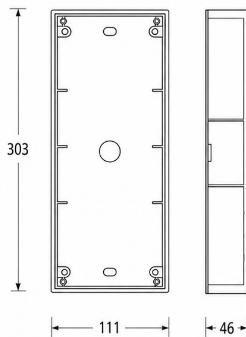
PUSZKA MONTAŻOWA (czarna)
